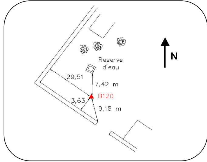
Croquis
